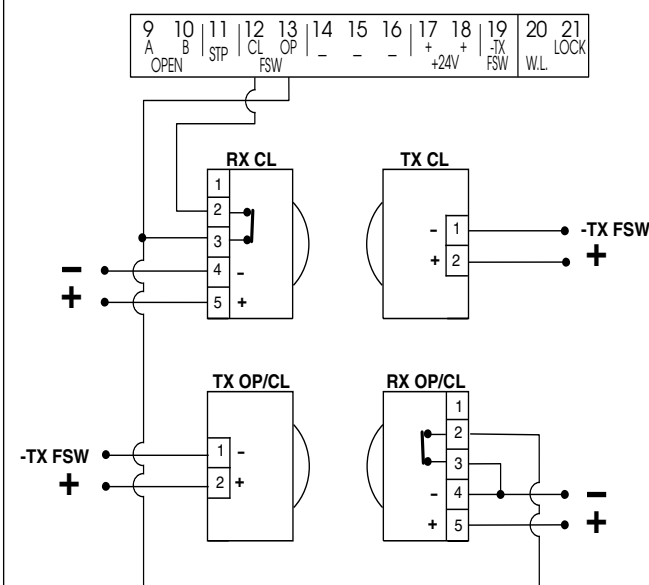
Connexion d'une paire de photocellules en fermeture, et d'une paire de photocellules en ouverture/fermeture (schéma préconisé)
