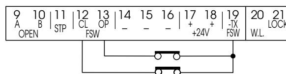
Connexion d'un dispositif de sécurité en fermeture et d'un dispositif de sécurité en ouverture
