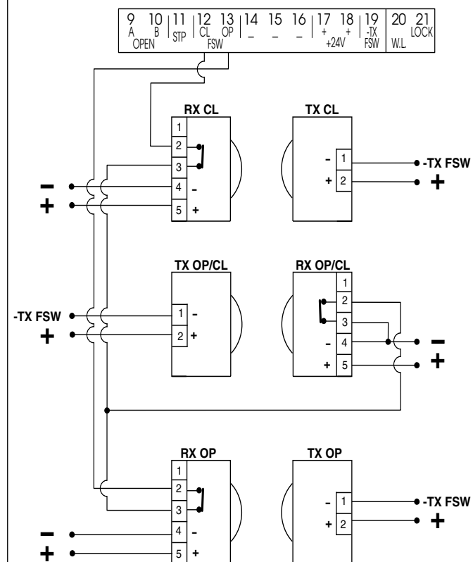
Connexion d'une paire de photocellules en fermeture, d'une paire de photocellules en ouverture et d'une paire de photocellules en ouverture/fermeture (schéma préconisé)
