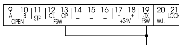
Connexion d'aucun dispositif de sécurité
