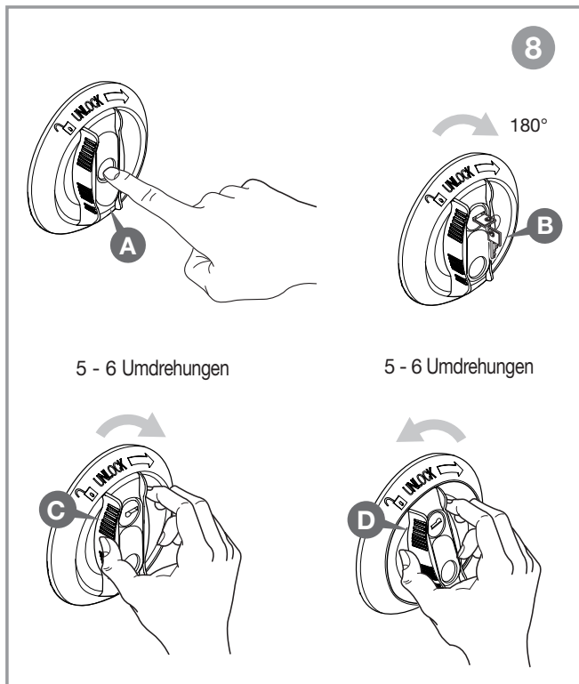
Entriegelungsverfahren (Abb. 8)
